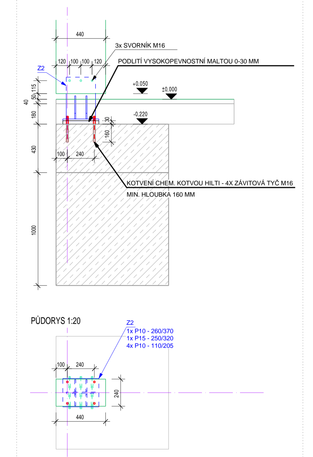
DET.2 - ŘEZ 1:20 - 8x
