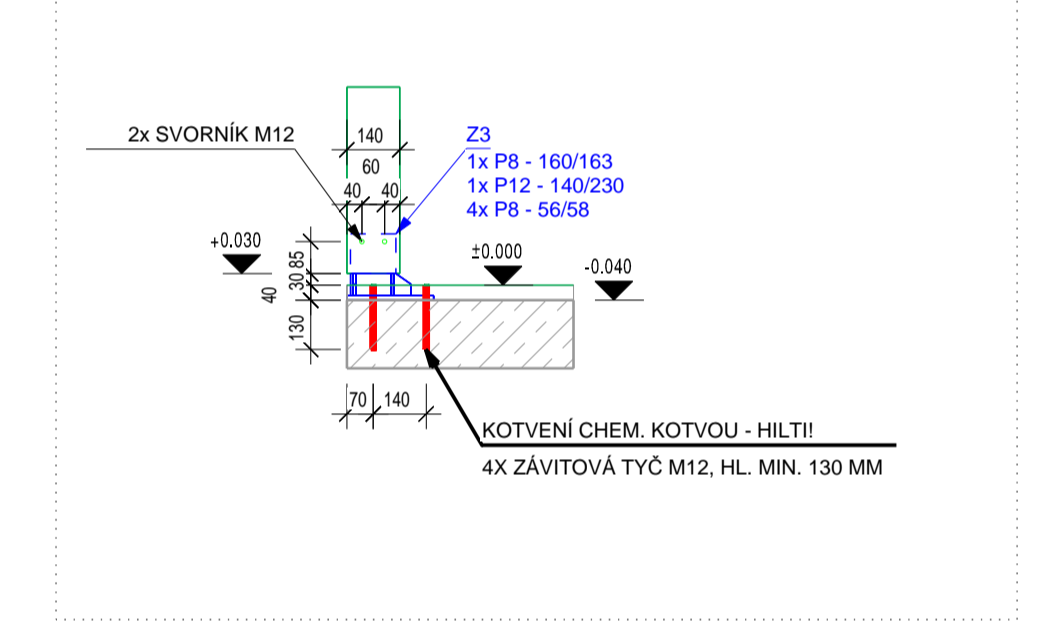
DET.3 - ŘEZ 1:20 - 5x
