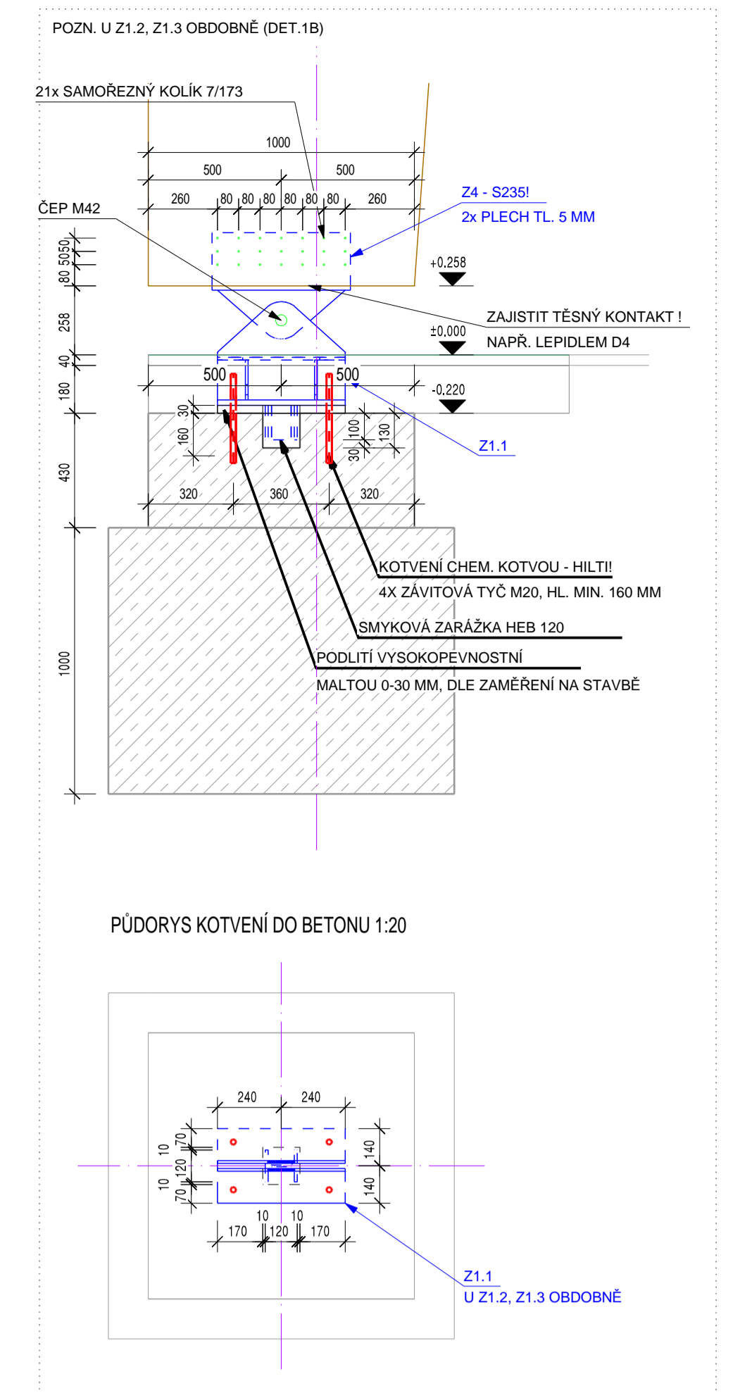
DET.2 - ŘEZ 1:20 - 8x
