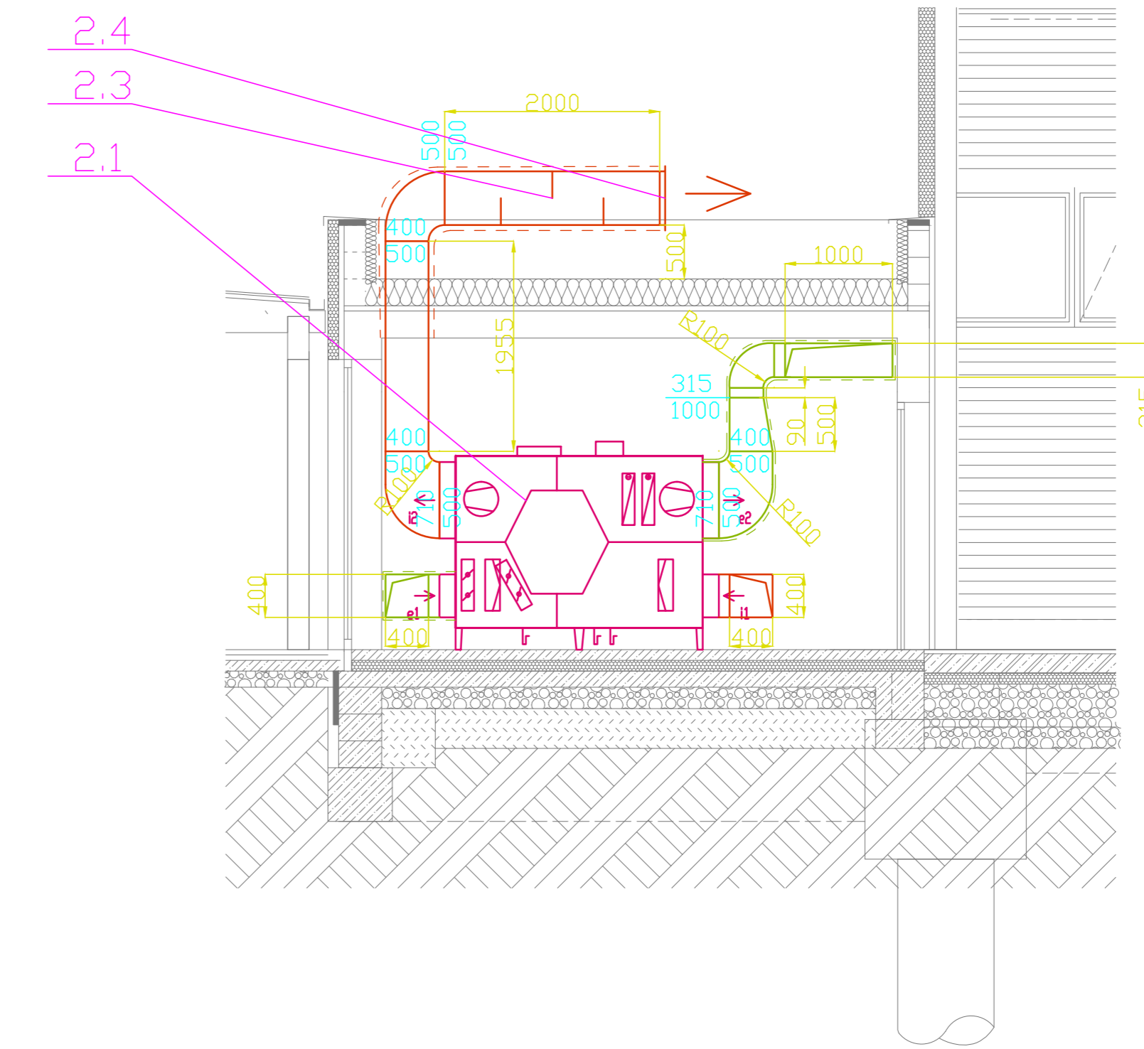
Rez strojovňou - zariadenie č. 2
