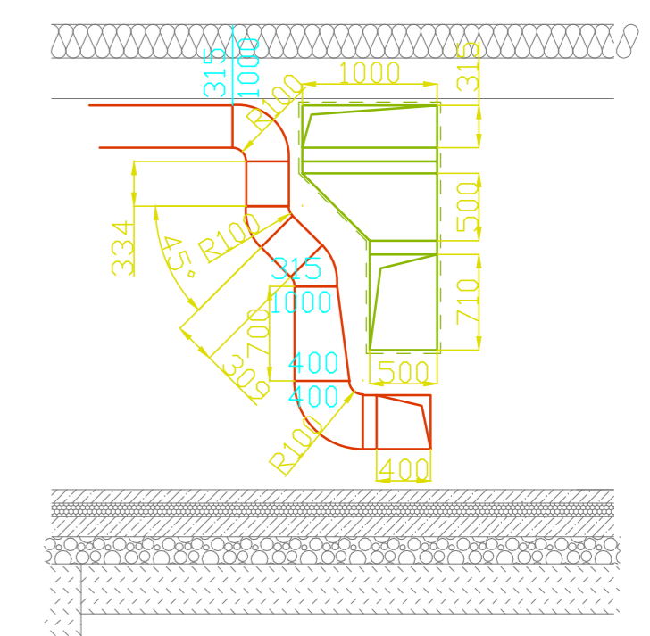
Zariadenie č. 2 - interiér
