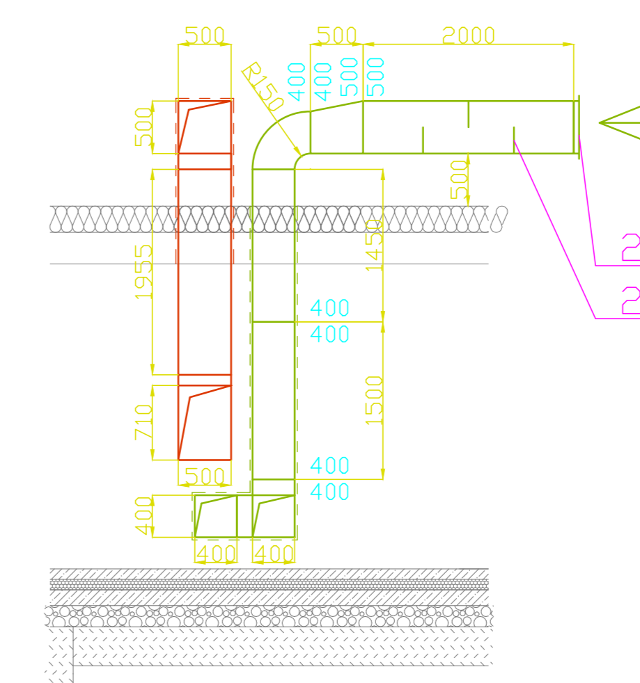
Zariadenie č. 2 - exteriér
